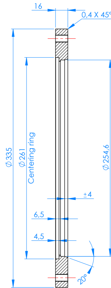
SECTION A-A
